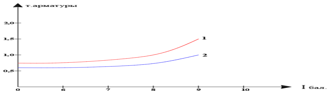
Расми 2. (а,б,в). Нишондиҳандаҳои техникӣ-иқтисодии хароҷоти мавод ба як метри тӯлонӣ гузаргоҳи зеризаминӣ.
