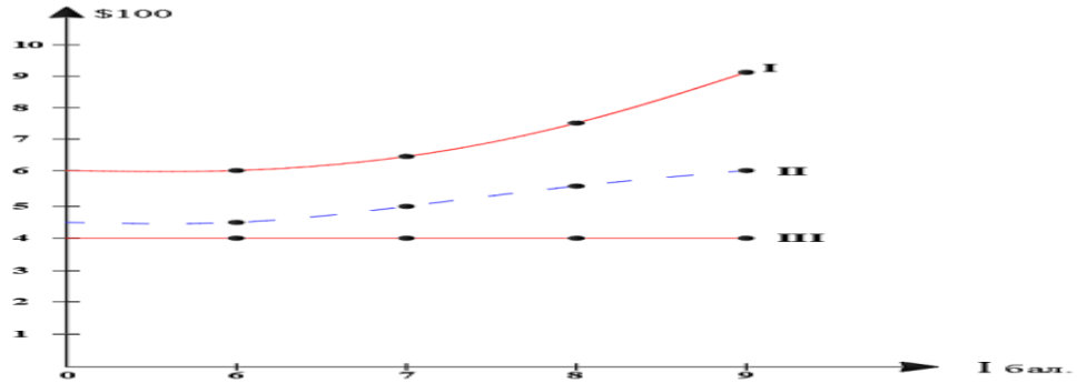
Расми 1. Арзиши иншоот ба як метри тӯлонӣ.
